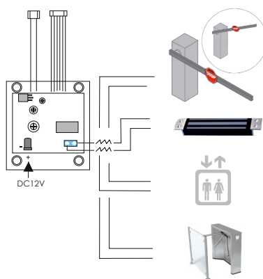
Esquema Eléctrico Esquema Eléctrico Electric Plan
